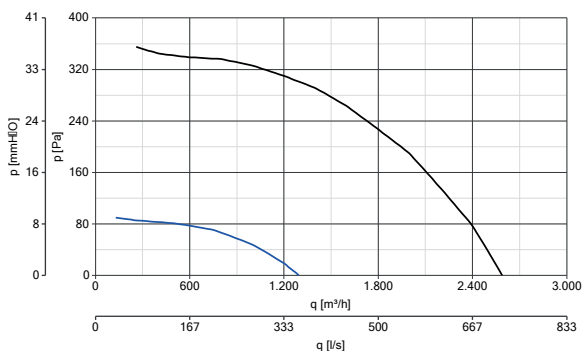
HEATMASTER F400 315 T4/8 0,25/0,03KW 120°C codice 15304
