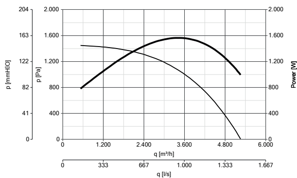
HEATMASTER F400 315 T2 1,5KW 80°C codice 15312
