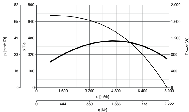
HEATMASTER F400 450 T4 1,1KW 120°C codice 15264
