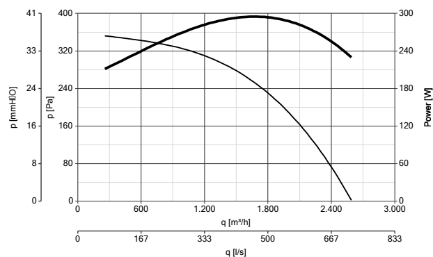
HEATMASTER F400 315 M4 0,25KW 80°C codice 15323
