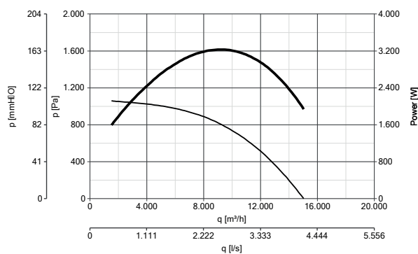
HEATMASTER F400 560 T4 3KW 120°C codice 15266
