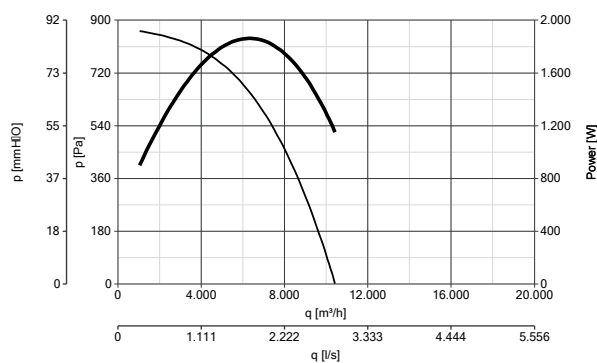
HEATMASTER F400 500 T4 1,5KW 120°C codice 15265
