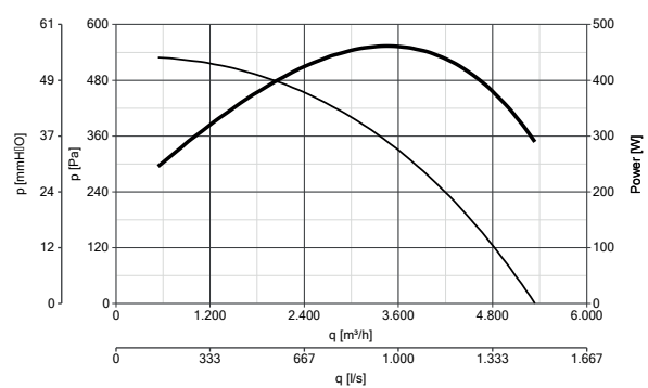
HEATMASTER F400 400 M4 0,55KW 120°C codice 15303
