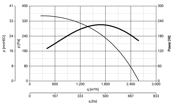
HEATMASTER F400 315 T4 0,25KW 120°C codice 15261
