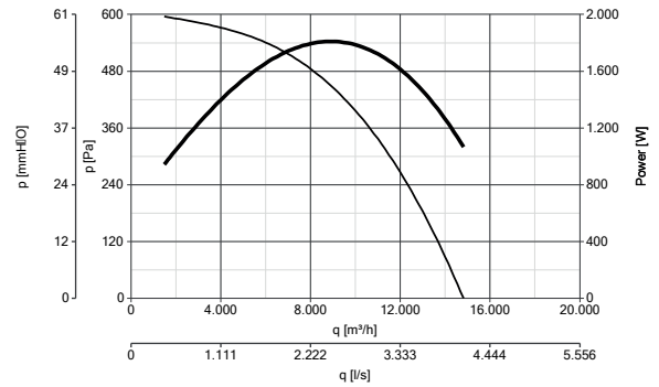
HEATMASTER F400 630 T6 1,5KW 80°C codice 15322
