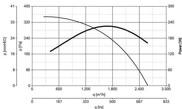
HEATMASTER F400 315 T4 0,25KW 80°C codice 15313
