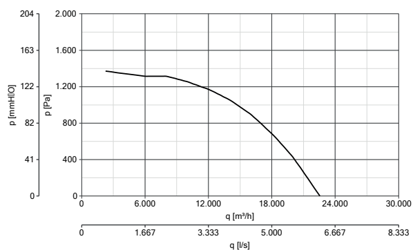
HEATMASTER F400 630 T4/8 5,5/1,1KW 120°C codice 15310
