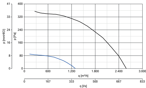
HEATMASTER F400 315 T4/8 0,25/0,03KW 80°C codice 15326
