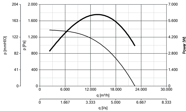
HEATMASTER F400 630 T4 5,5KW 80°C codice 15319
