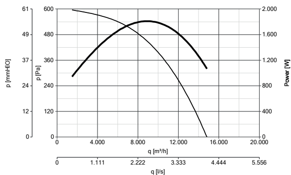
HEATMASTER F400 630 T6 1,5KW 120°C codice 15270
