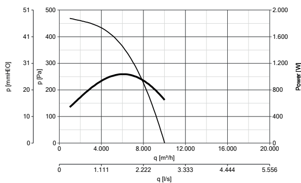
HEATMASTER F400 560 T6 1,1KW 120°C codice 15269
