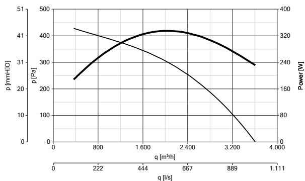
HEATMASTER F400 355 T4 0,25KW 120°C codice 15262
