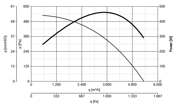
HEATMASTER F400 400 M4 0,55KW 80°C codice 15325
