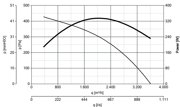
HEATMASTER F400 355 T4 0,25KW 80°C codice 15314
