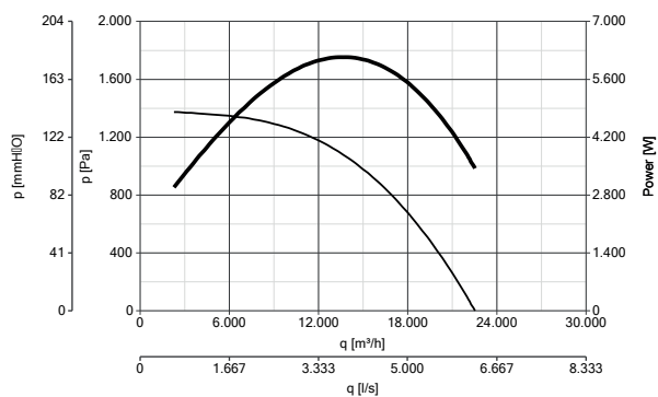
HEATMASTER F400 630 T4 5,5KW 120°C codice 15267
