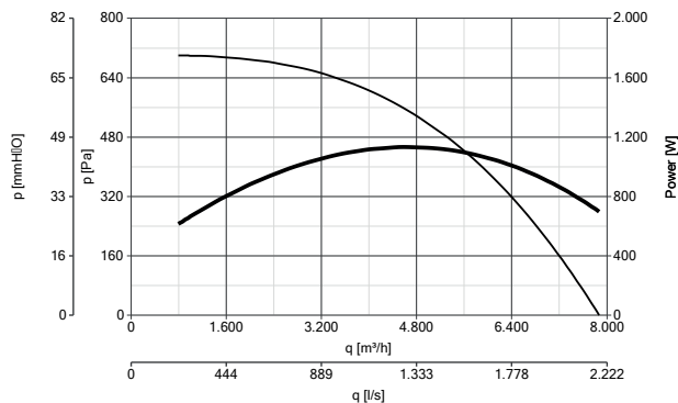
HEATMASTER F400 450 T4 1,1KW 80°C codice 15316
