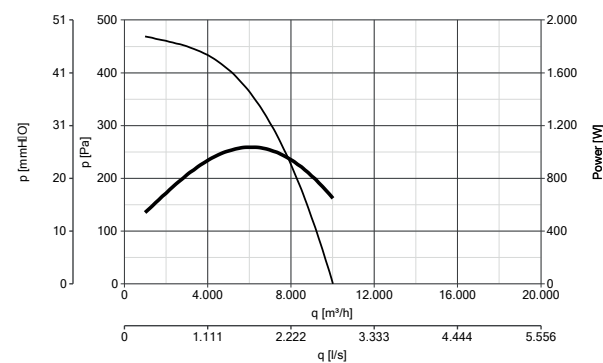
HEATMASTER F400 560 T6 1,1KW 80°C codice 15321
