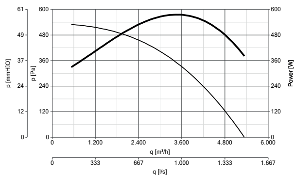
HEATMASTER F400 400 T4 0,55KW 120°C codice 15263
